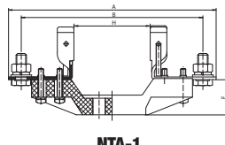
NTA-1
