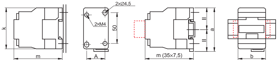
Montage auf Montageplatte
