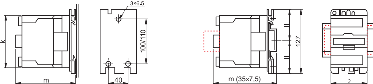
Montage auf Montageplatte
