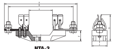
NTA-3
