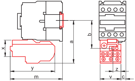
TR2HD1..
