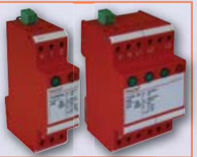
Parafoudres de type 3 (protection "fine"), version modulaire 6
