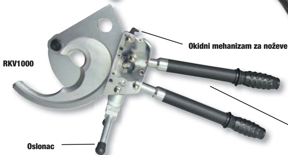
Drška sa teleskopom
